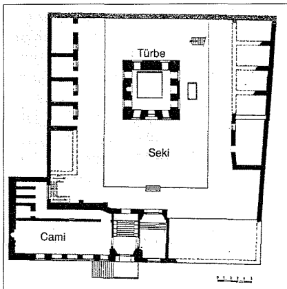
İbrâhim Gülşeni Külliyesi'nin planı
